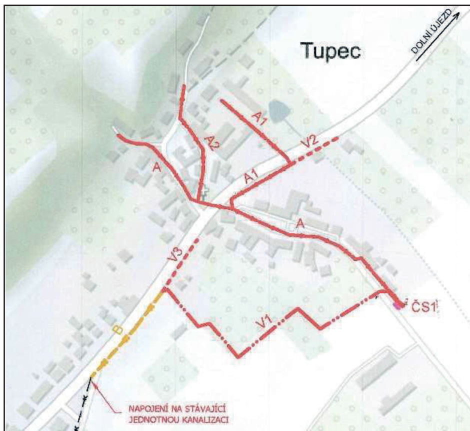
Výkres plánované stavby kanalizace Tupec
